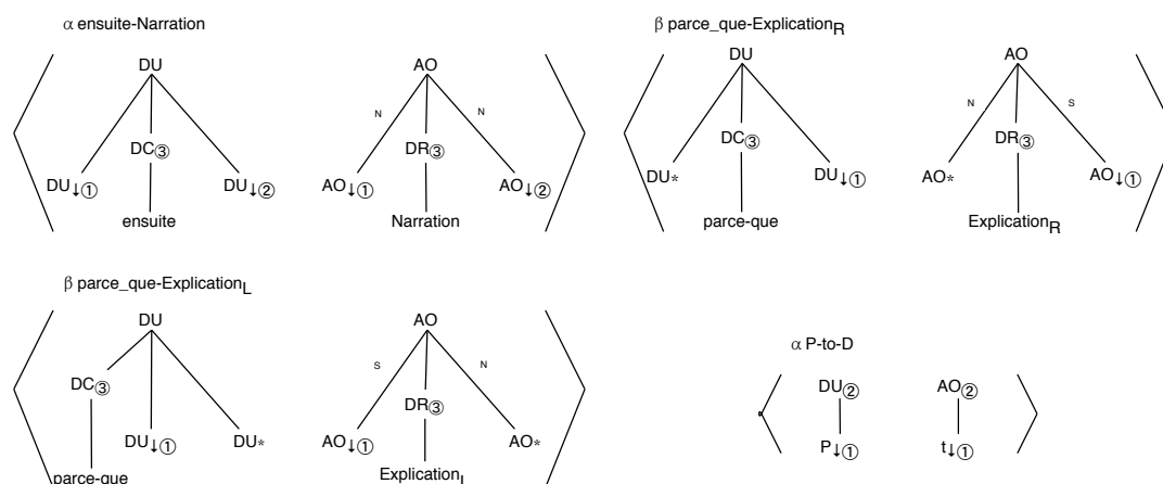
FIG. 4 – Fragment d'une grammaire D-STAG pour le français
