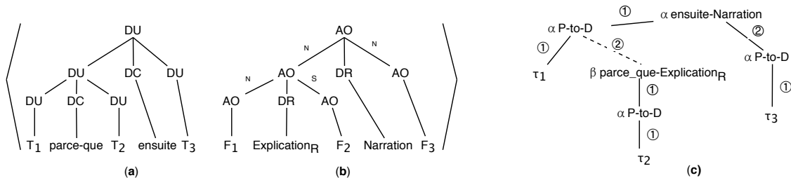
FIG. 5 – Paire d’arbres dérivés (a)-(b) et arbre de dérivation (c) calculés en D-STAG pour (1)
